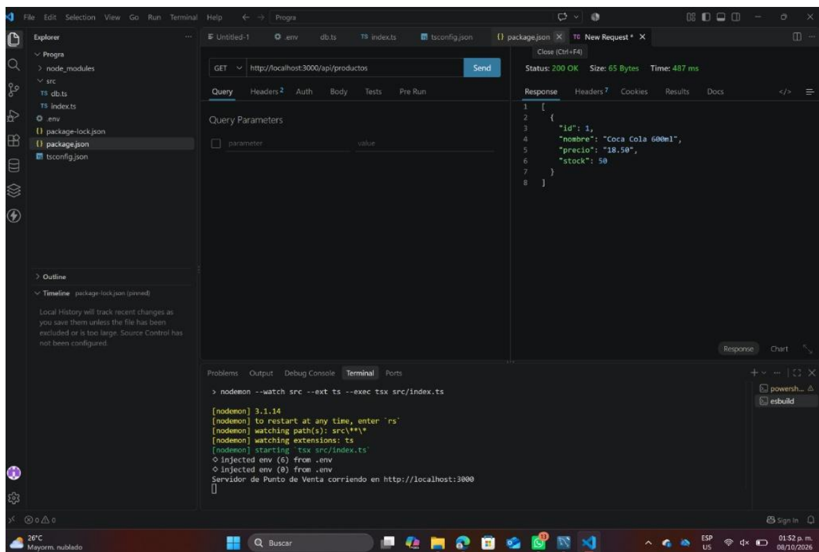
Figura 1: Servidor Node.js activo y respondiendo a la ruta /api/productos.
